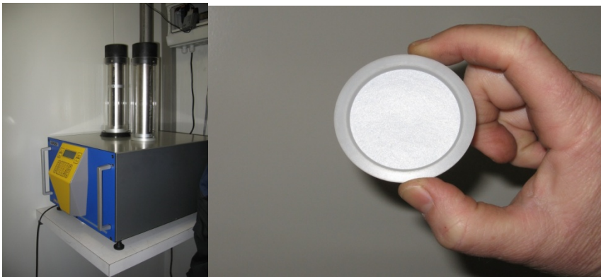
Exempel på mätinstrument för partikelhalter, SM200 med filterkassetter och filter
